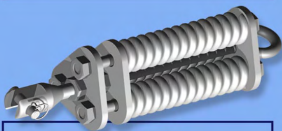
articolo "AM" AMMORTIZZATORE IN ACCIAIO INOX Permette l'assorbimento dell'energia in caso di caduta.
