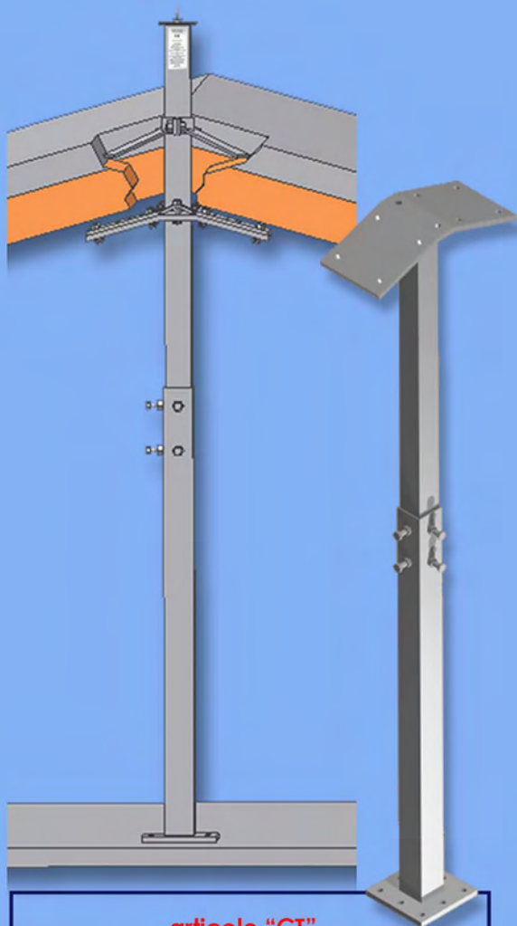
articolo "CT" COLONNA TELESCOPICA IN ACCIAIO PER TETTO IN MURICCI E TAVELLONI
