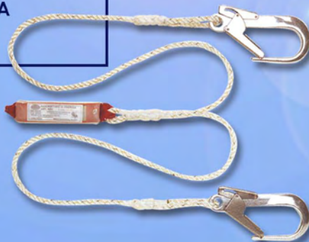
articolo "CDSR" FUNDE MARLOW A TRE TREFOLI Ø 16 - LUNGHEZZA 10 / 20 / 30 mt
